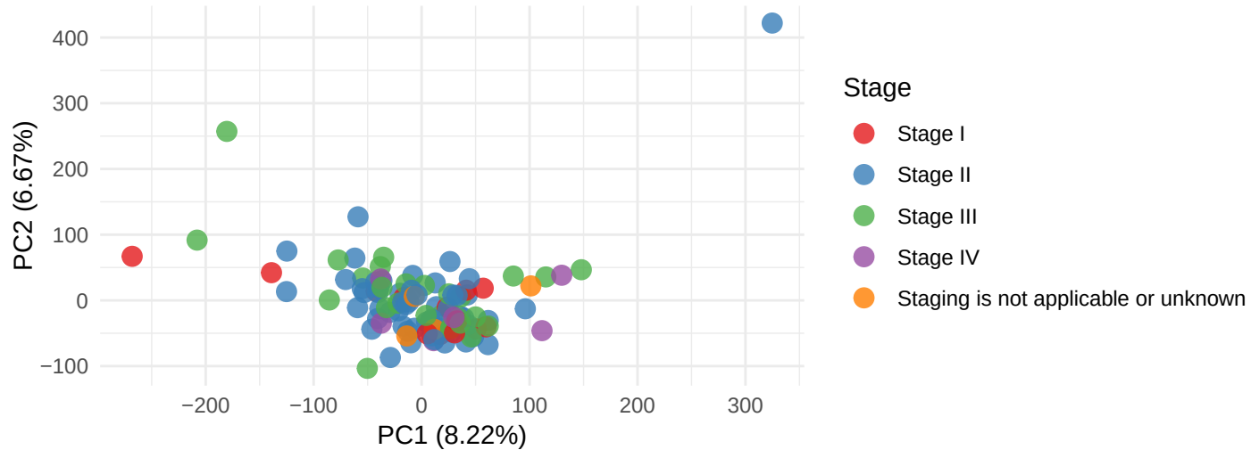
PCA: CNV Layer
